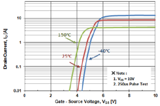
Fig. 2 I_D - V_{GS}
