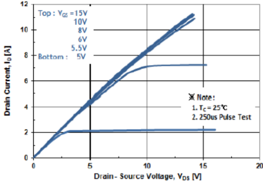
Fig. 1 I_D - V_{DS}
