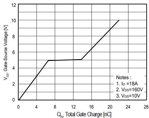
Fig. 6 V_{GS} - Q_G
