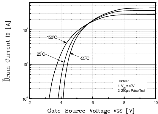
Fig. 2 I_D - V_{GS}
