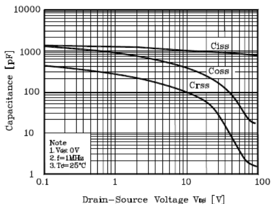
Fig. 5 Capacitance - V_{DS}
