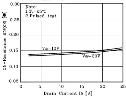
Fig. 3 R_{DS(on)} - I_D
