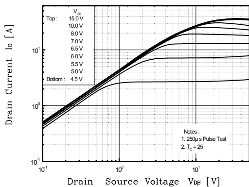
Fig. 1 I_D - V_{DS}
