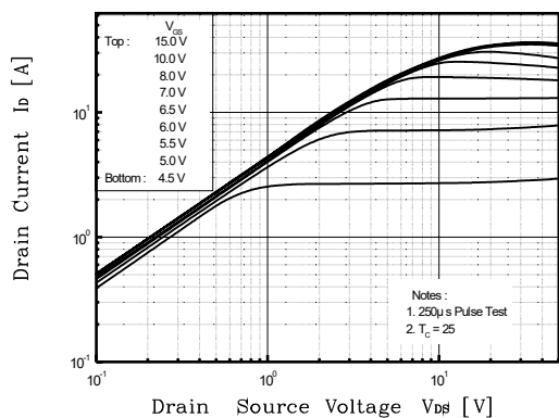
Fig. 1 I_D - V_{DS}
