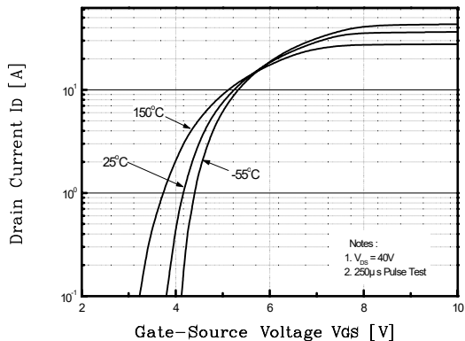
Fig. 2 I_D - V_{GS}
