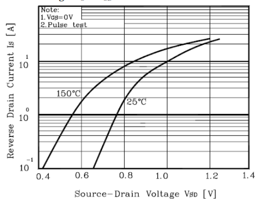
Fig. 4 I_S - V_{SD}
