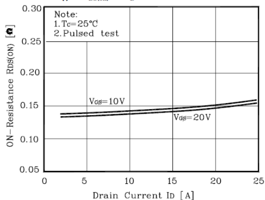
Fig. 3 R_{DS(on)} - I_D
