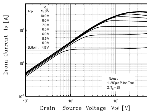
Fig. 1 I_D - V_{DS}
