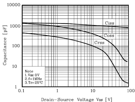
Fig. 5 Capacitance - V_{DS}
