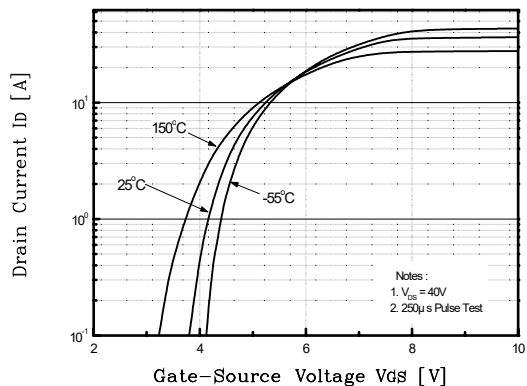
Fig. 2 I_D - V_{GS}
