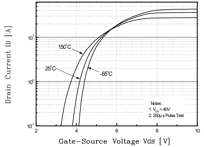
Fig. 2 I_D - V_{GS}
