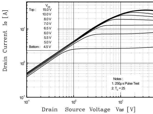
Fig. 1 I_D - V_{DS}
