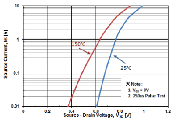
Fig. 4 I_S - V_{SD}
