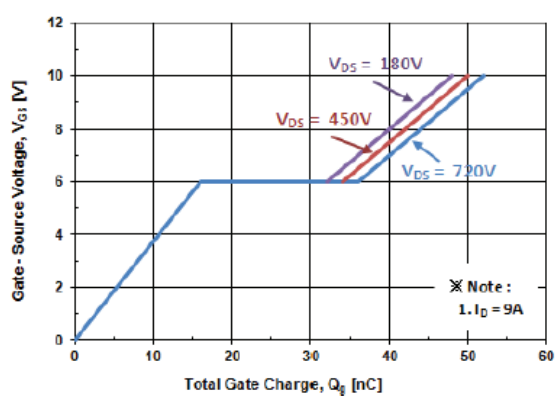
Fig. 6 V_{GS} - Q_G
