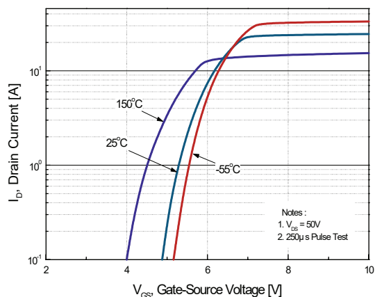
Fig. 2 I_D - V_{GS}
