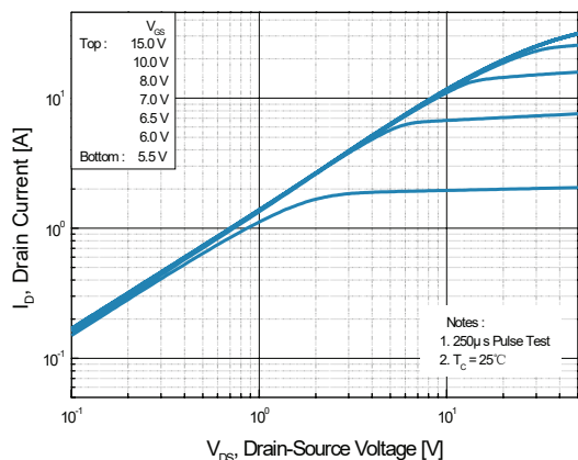
Fig. 1 I_D - V_{DS}
