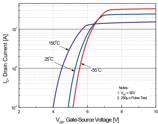
Fig. 2 I_D - V_{GS}
